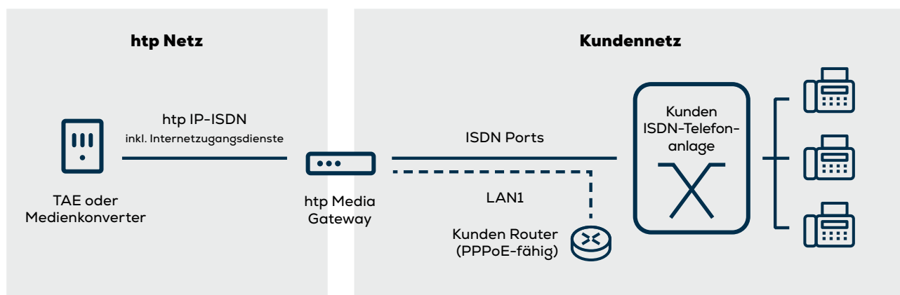
Abb.: IP-ISDN Kundenanschlussschaltung unter Verwendung eines kundeneigenen Routers
